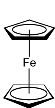
Ferrocene staggered
