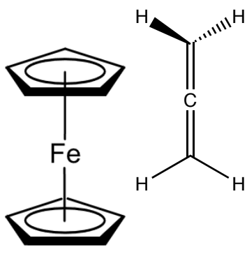
Ferrocene eclipsed
