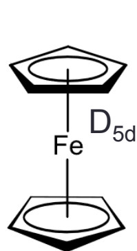
Ferrocene staggered
