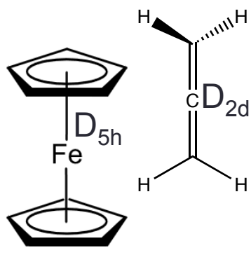
Ferrocene eclipsed
